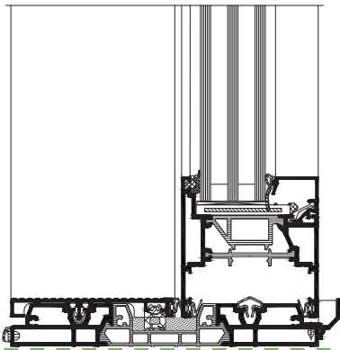
Soglia ribassata 25 mm Versione a una, due e tre rotaie Ideale per la ristrutturazione
